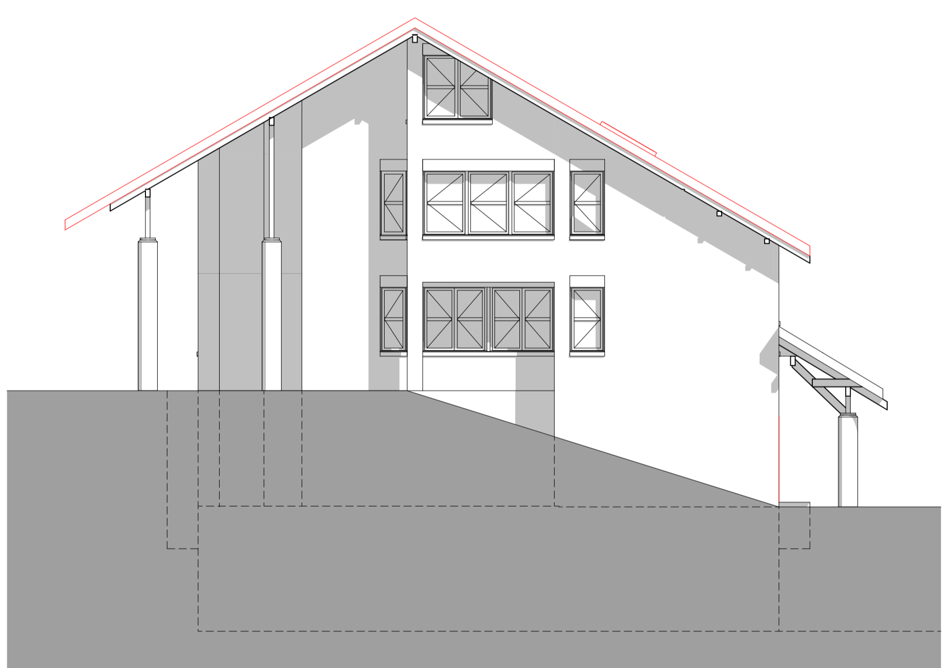
Nordwestfassade Gemeindehaus
