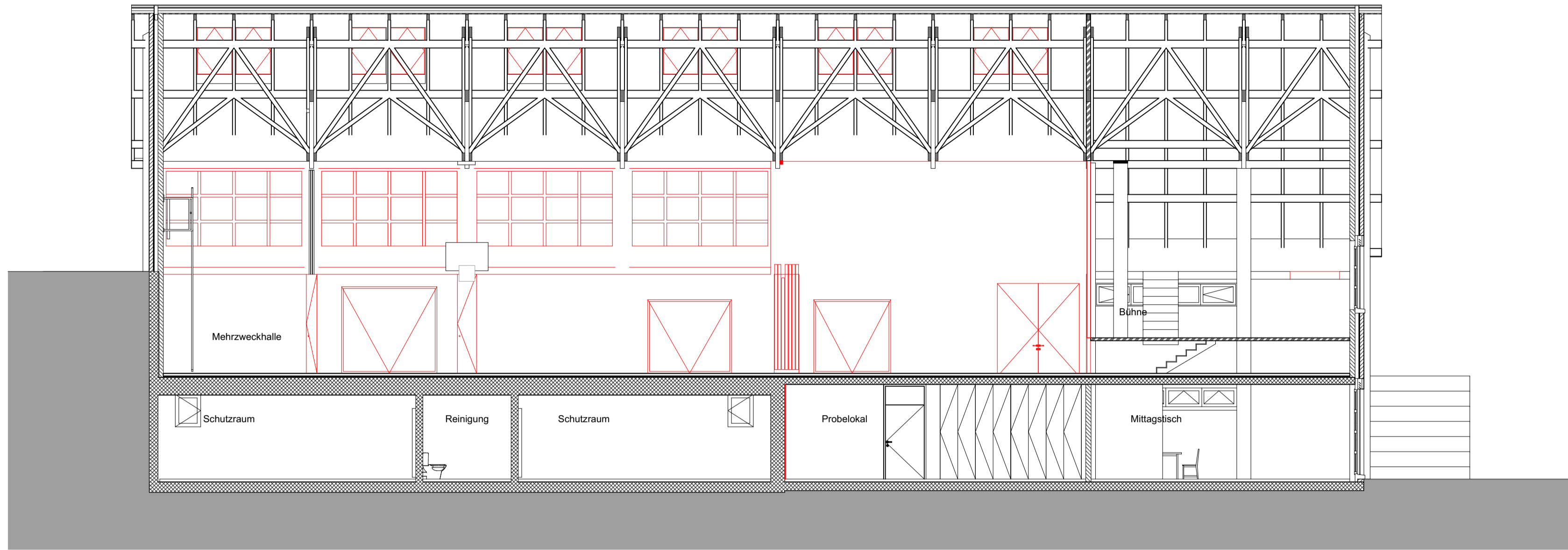
Schnitt D Turnhalle
