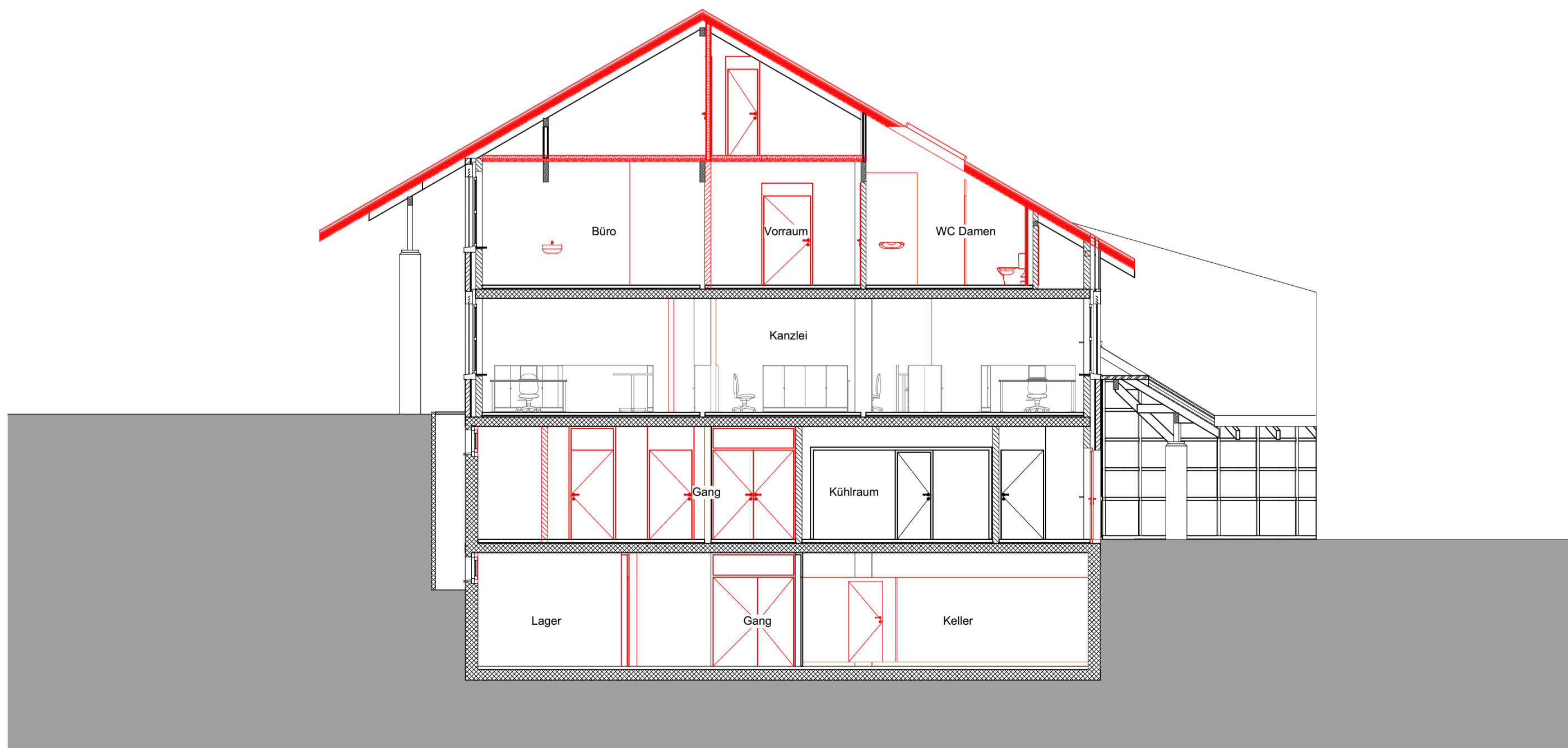
Schnitt C Gemeindehaus
