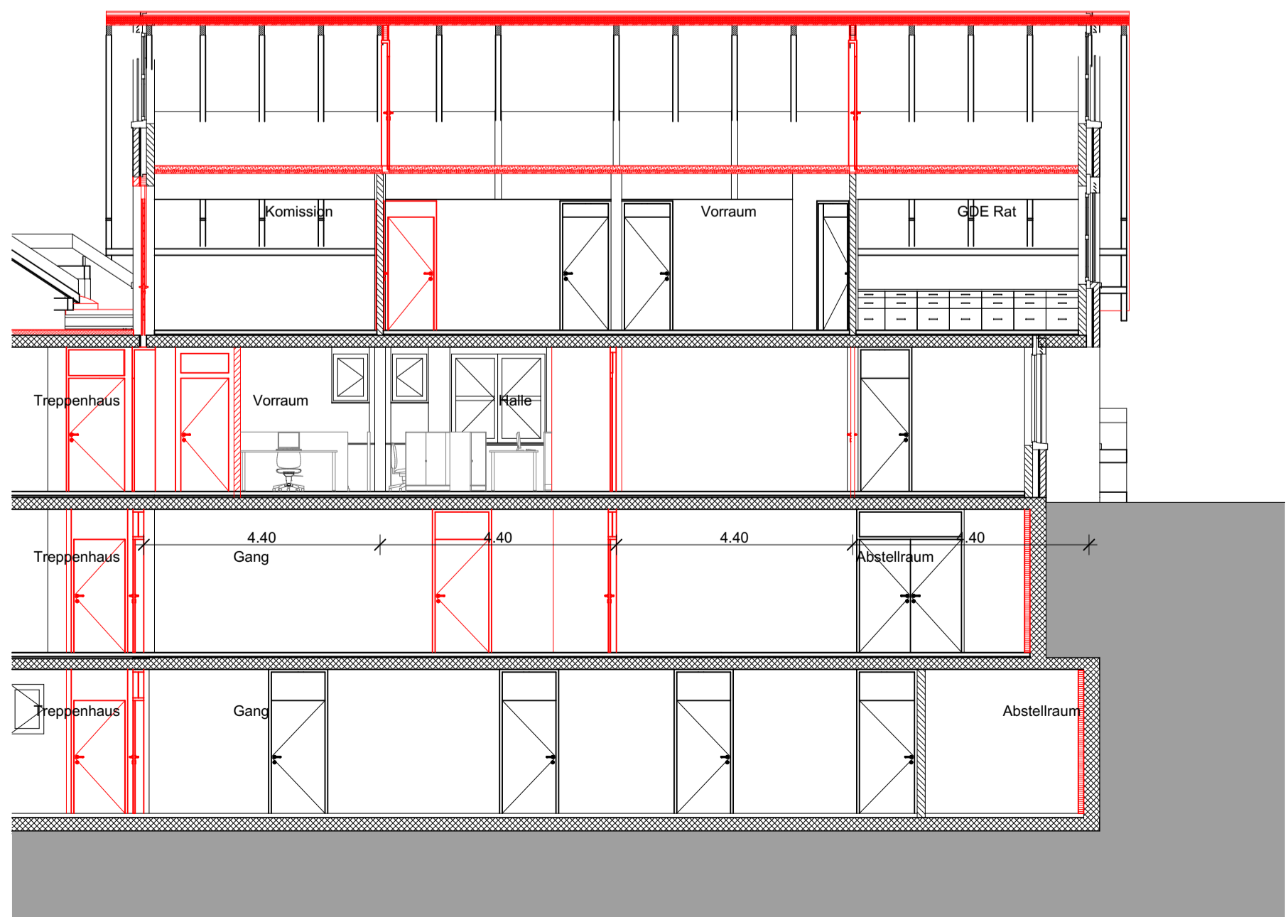
Schnitt E Gemeindehaus
