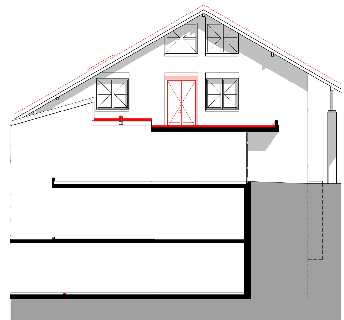
Südostfassade Gemeindehaus
