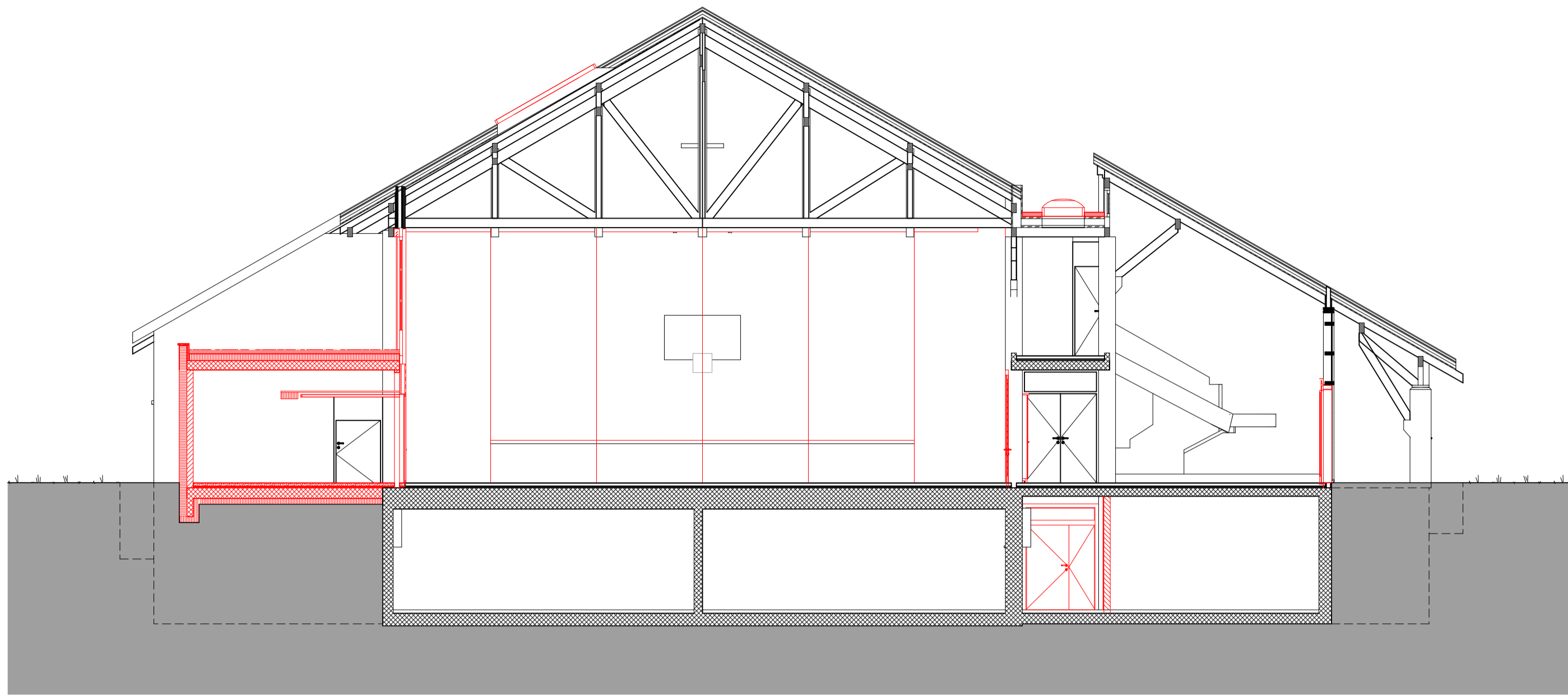
Schnitt A Turnhalle
