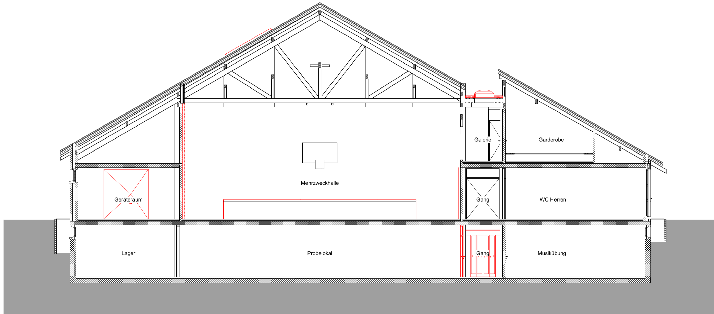
Schnitt B Turnhalle
