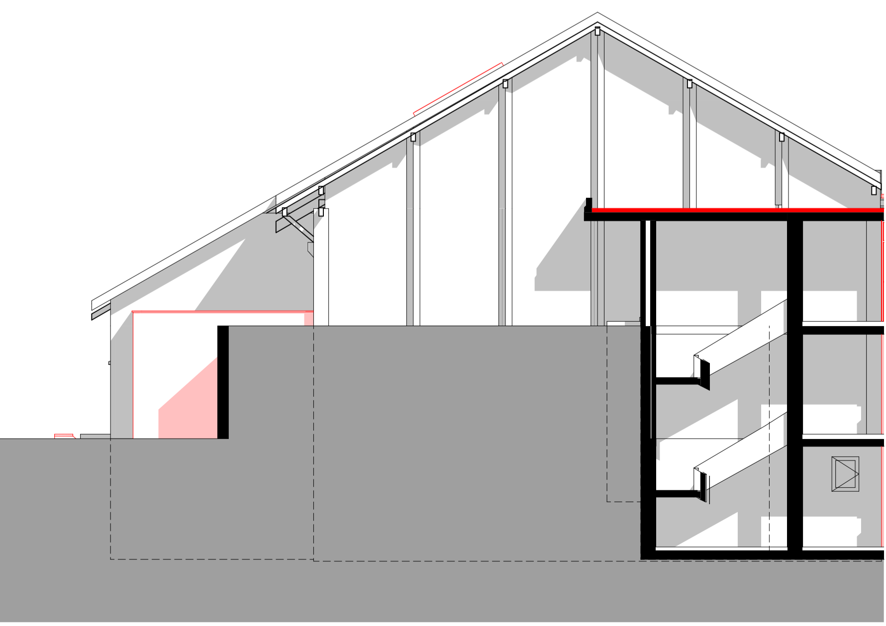
Nordfassade Turnhalle
